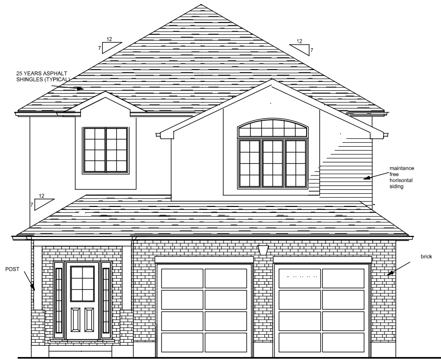
elevation A
